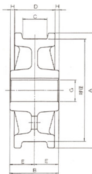
NR-B型 (車輪踏面巾C-80)
