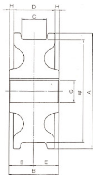
NR-A型 (車輪踏面巾C-60)
